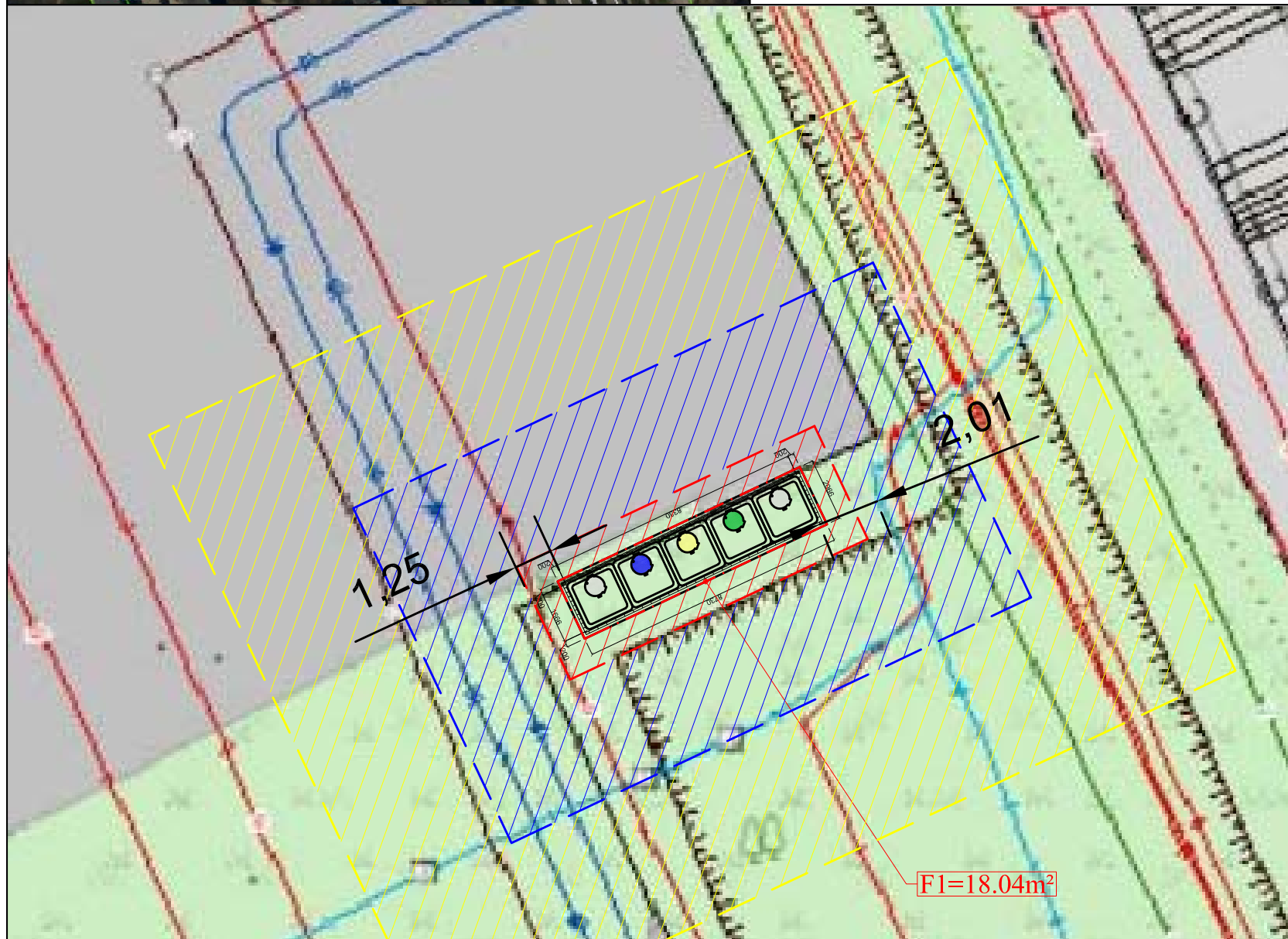
Pusiau požeminių konteinerių aikštelės schema Nr.: 2, M 1:50
