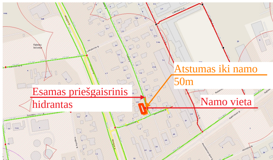
Pav. 1. Priešgaisrinių hidrantų schema
