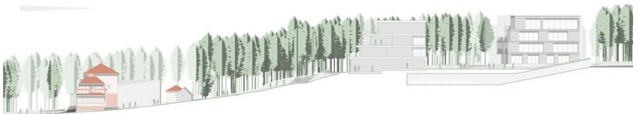
13 pav. Teritorijos pjūvis vakarų-rytų kryptimi ties Luizės pastatų kompleksu
