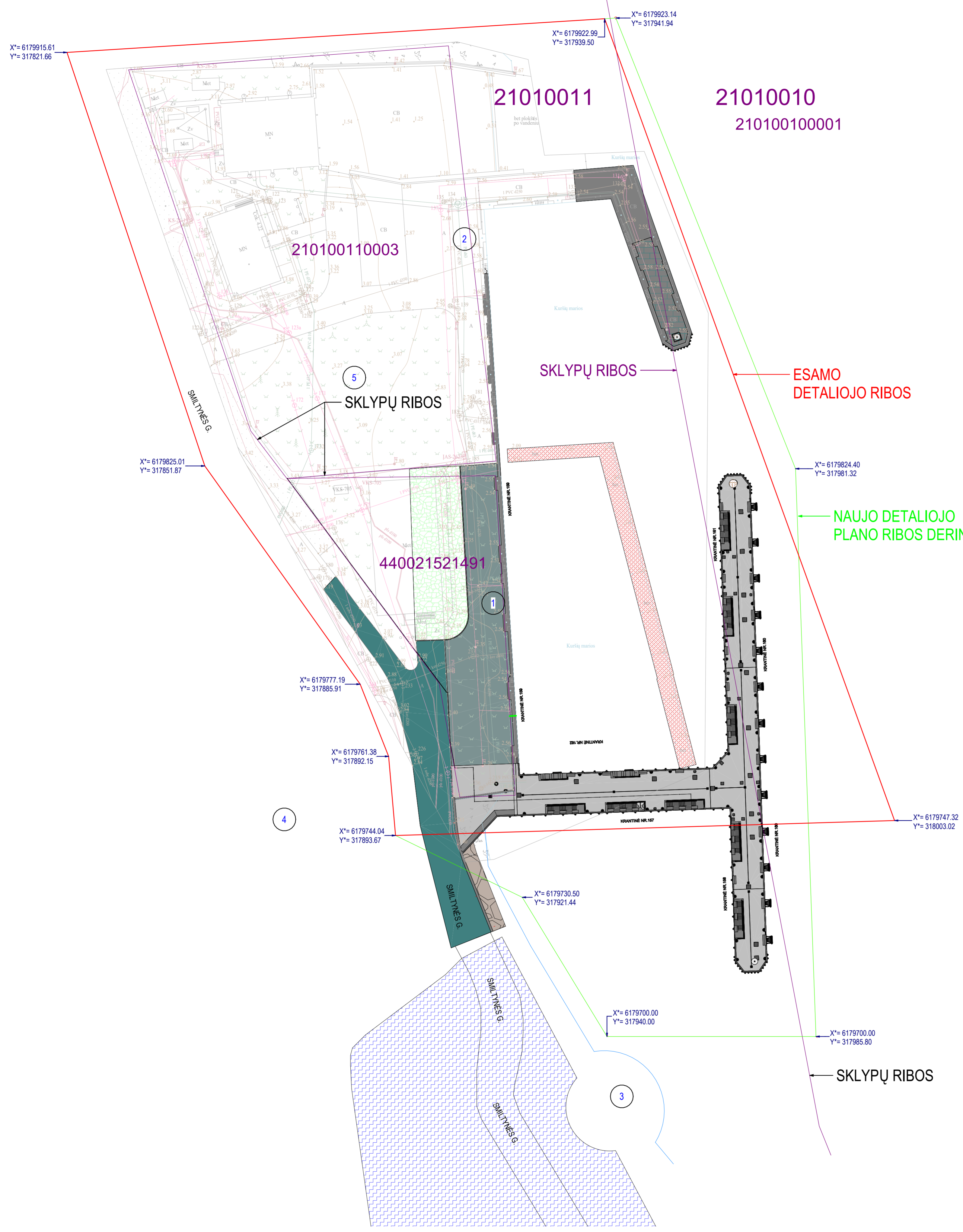
1 SITUACIJOS PLANAS M 1 : 500
