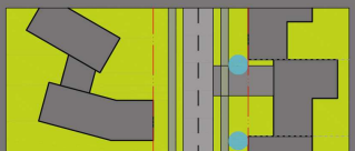
GYVENAMOJO KVARTALO GATVĖS PJŪVIS IR SCHEMA M 1:500
